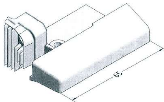
Tappo montante cieco (apertura interna) RAL 704
